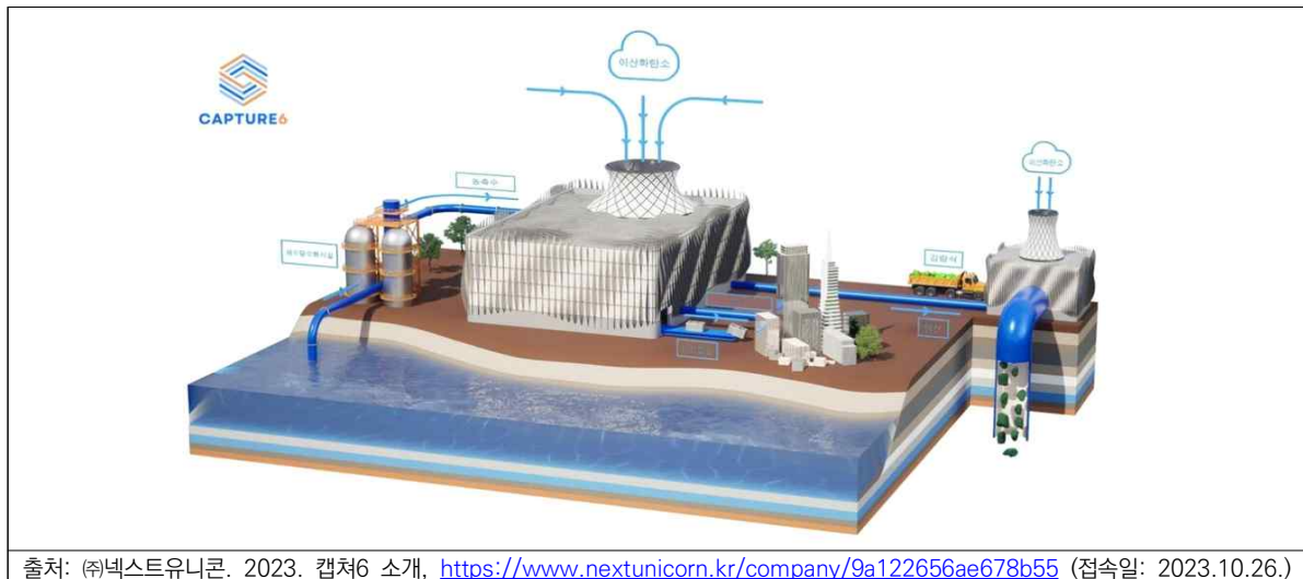
[그림 2-3-11] 습식 탄소포집 시설
